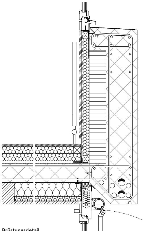
Brüstungsdetail
