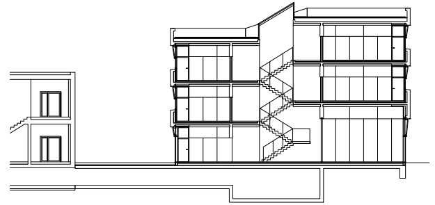
Querschnitt
